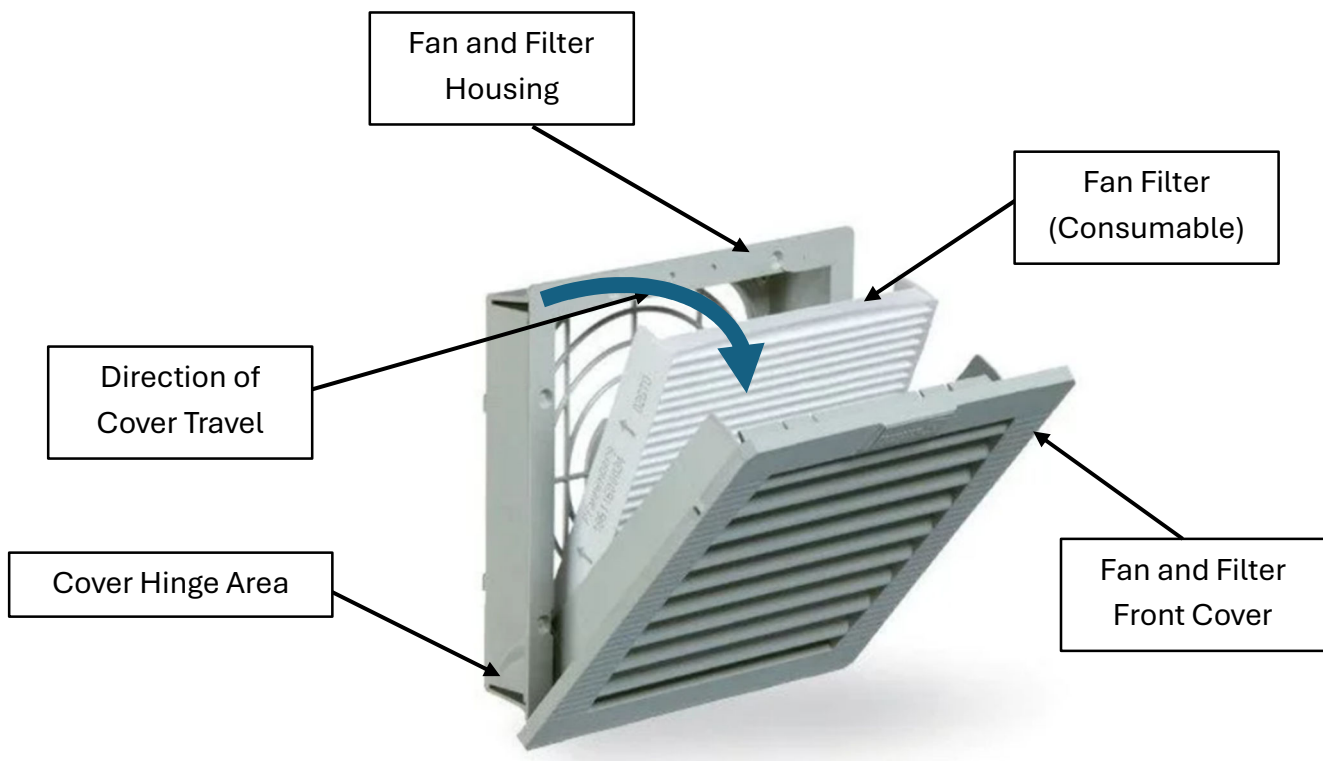
Fan Filter Access
